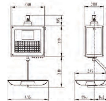
CE 9900 EVO
