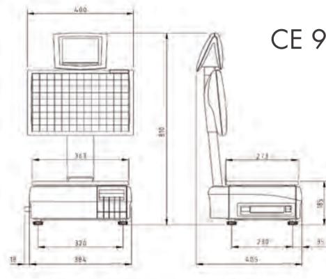
CE 9900 EVO
